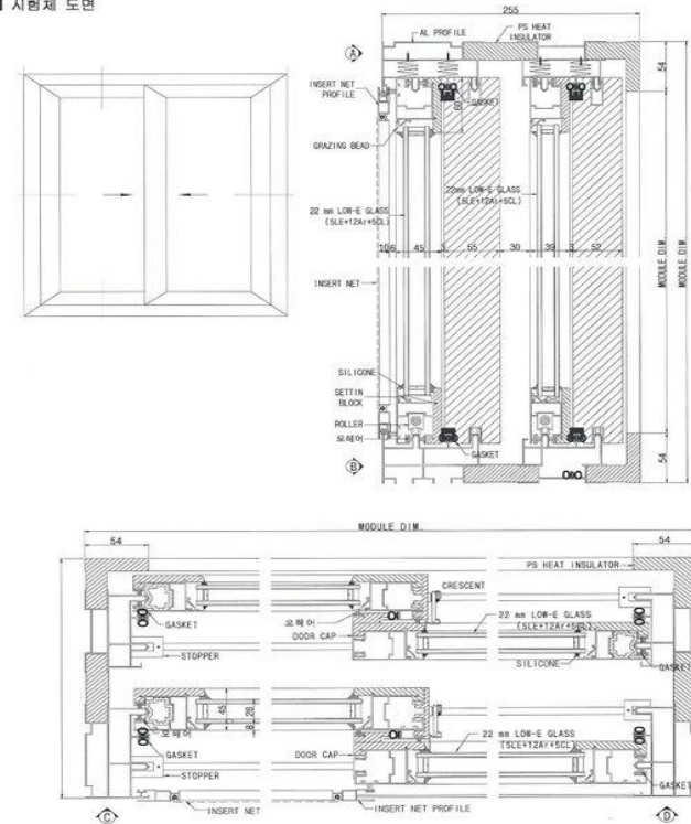
□ 시험체 입면도 및 단면도
